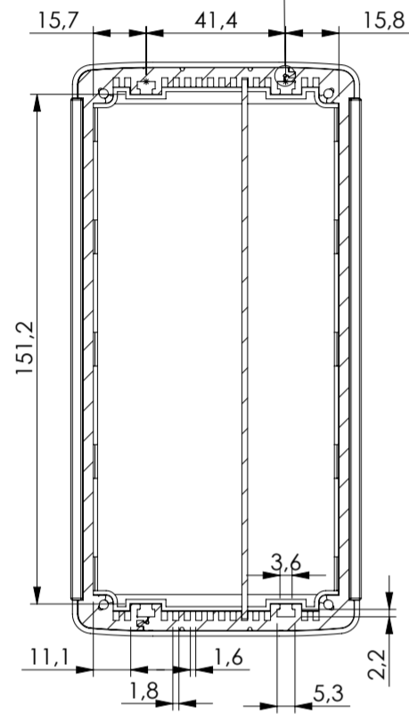
SEZIONE B-B
